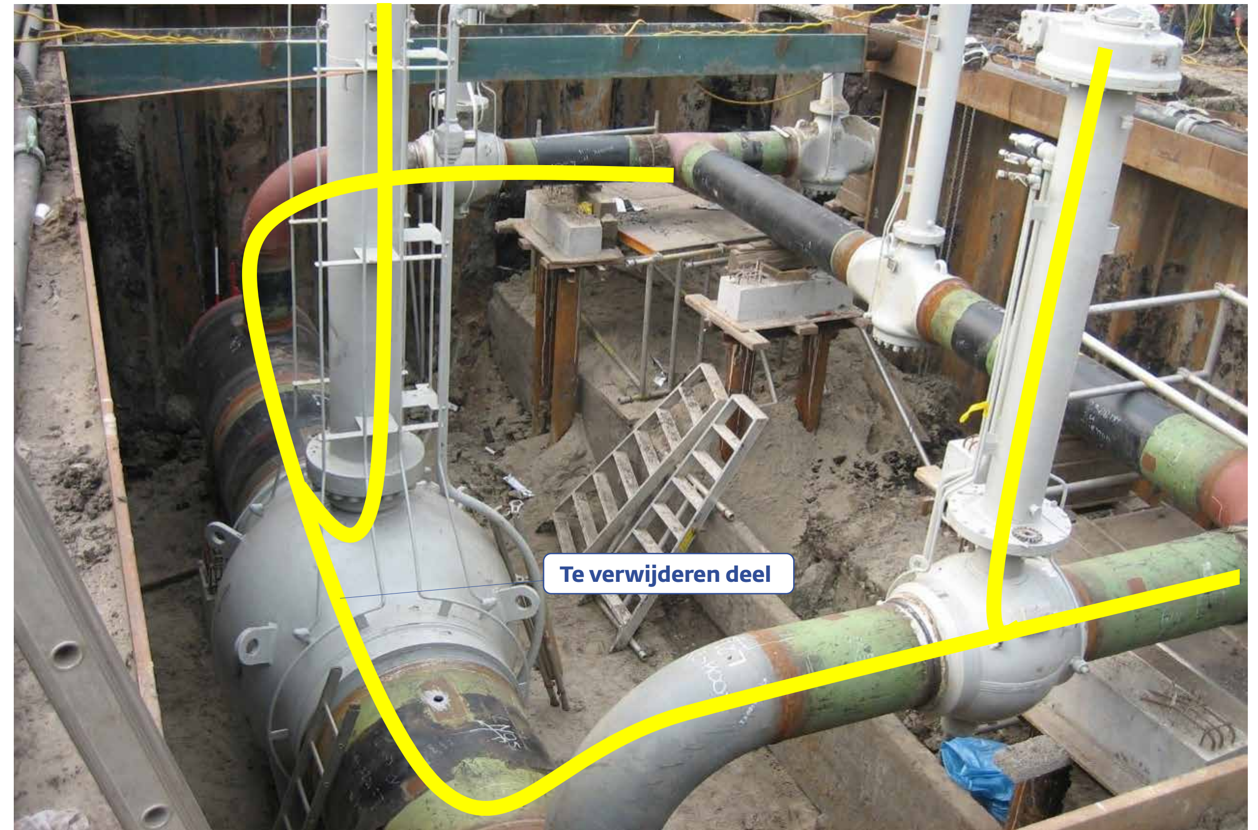
Afsluiterschema ondergronds
