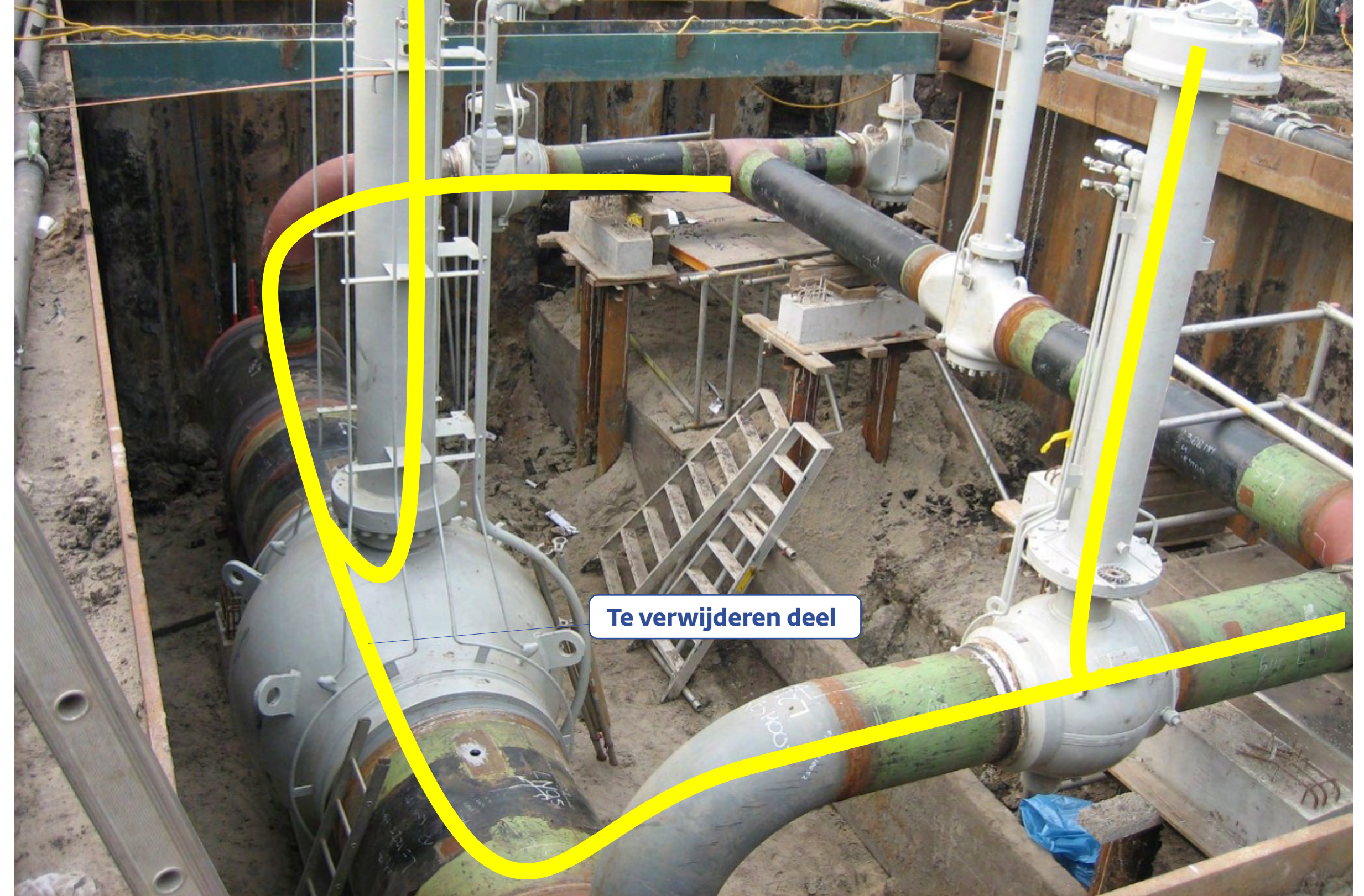
Afsluiterschema ondergronds
